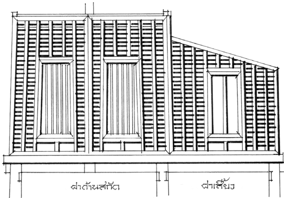
ฝาสำรวจไม้จริง
