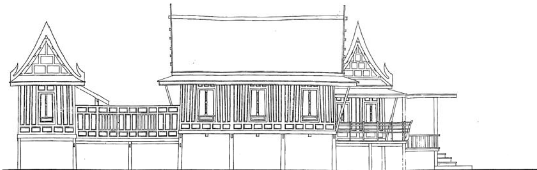
รูปปั้นด้านข้างของหมู่เจ็ด (เขียนแบบ)
