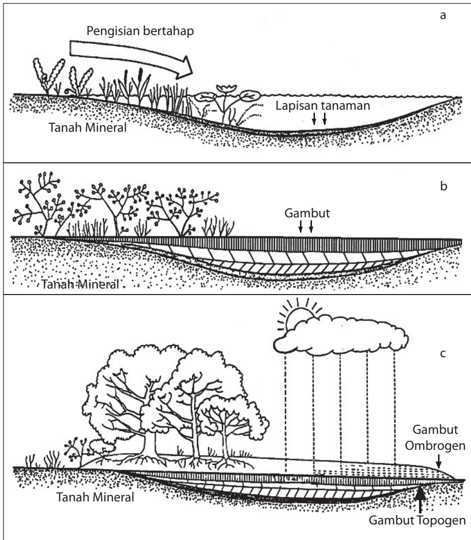
Gambar 1. Skema proses pembentukan dan perkembangan ketebalan hampan gambut pada suatu cekungan lahan basah: a. Pengisian danau dangkal oleh vegetasi lahan basah, b. Pembentukan gambut topogen, dan c. Pembentukan kubah gambut ombrogen berada di atas gambut topogen (dari Noor, 2001 mengutip van de Meene, 1984).
