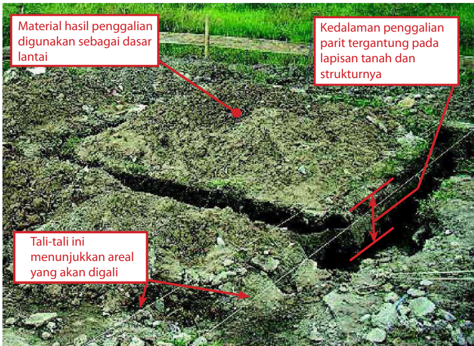
Parit-parit yang telah digali untuk pembuatan fondasi
