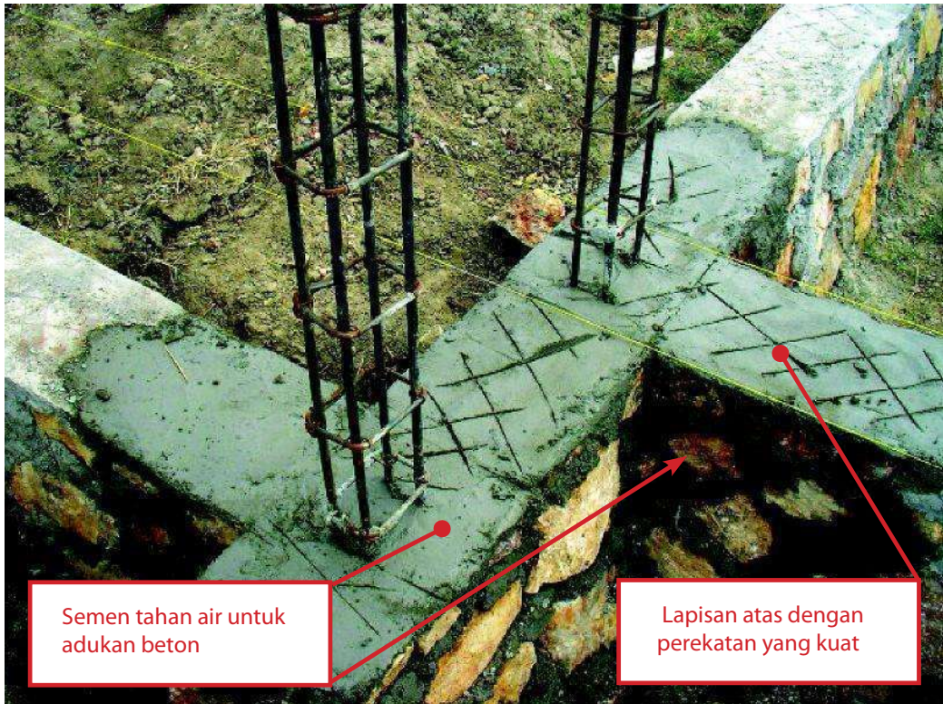
Fondasi menerus yang dibangun dengan baik
