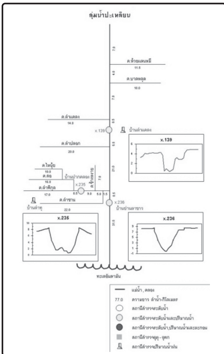
ภาพที่ 15 แผนผังแสดงสถานีสำรวจอุทกวิทยาลุ่มน้ำปะเหลียน
