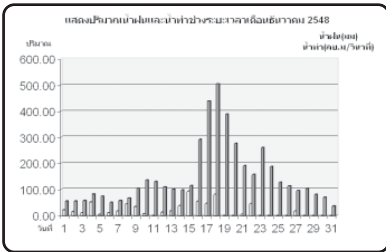
ภาพที่ 18 ปริมาณน้ำฝนและน้ำท่าที่สถานี x236 ช่วงเดือนธันวาคม 2548
