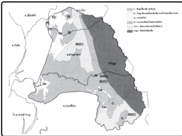
ภาพที่ 8 แสดงชั้นดินในเขตลุ่มน้ำสาขาลองปะเหลียน
