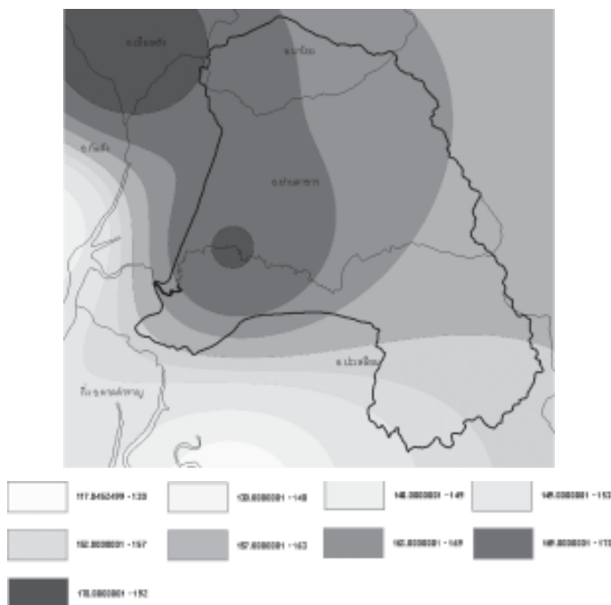
ภาพที่ 4 แสดงเส้นชั้นน้ำฝนในบริเวณลุ่มน้ำสาขาคลองปะเหลียนเฉลี่ยรายปี (มม.)
