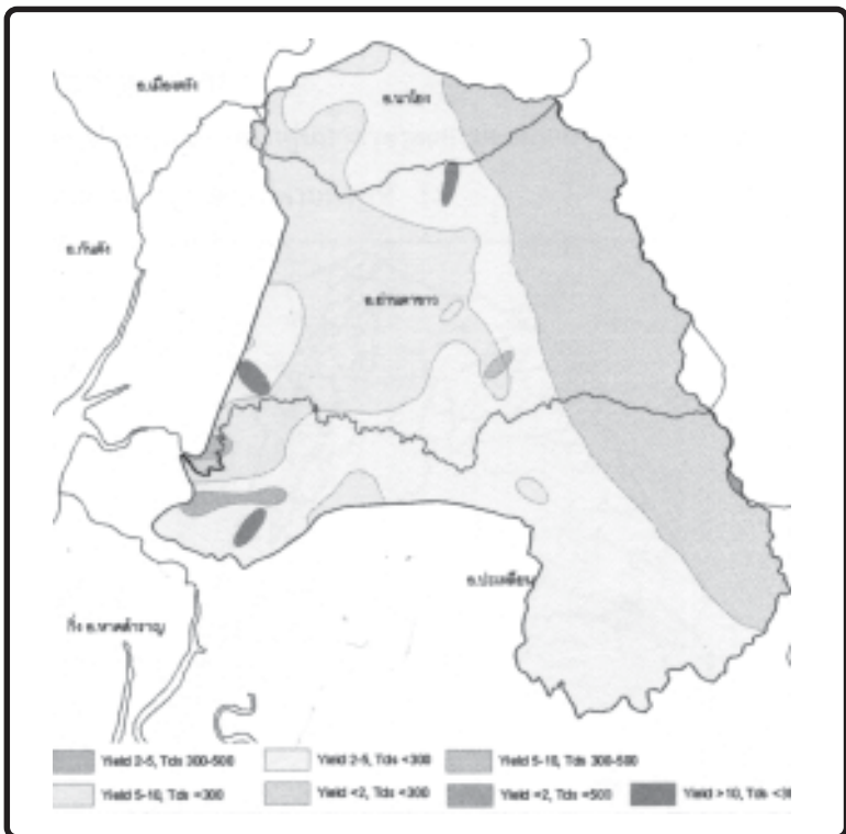
ภาพที่ 10 แสดงปริมาณน้ำบาดาลและปริมาณสารละลาย ในเขตลุ่มน้ำสาขาลองปะเหลียน
