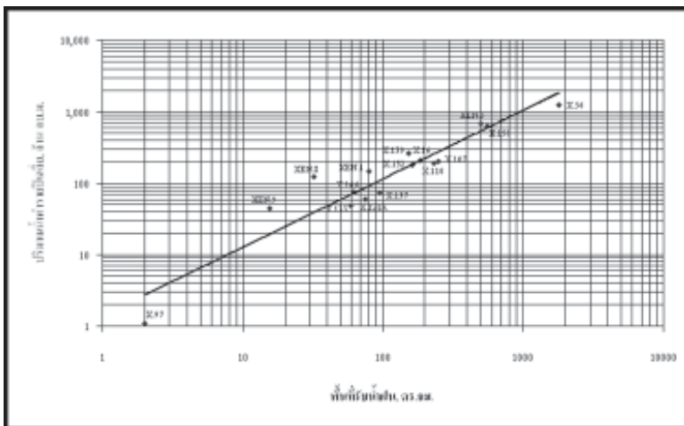
ภาพที่ 7 กราฟแสดงความสัมพันธ์ระหว่าง ปริมาณน้ำท่ารายปีเฉลี่ยและพื้นที่รับน้ำฝน
