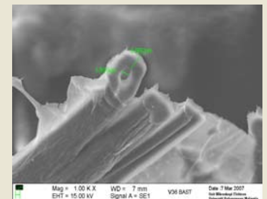
Mikrograf SEM menunjukkan gentian kenaf V36 SEM micrograph of Kenaf-V36 fibre
