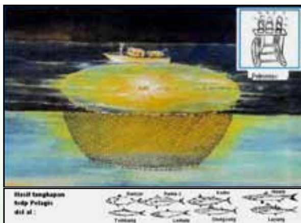
Pukat cincin dengan alat bantu lampu
